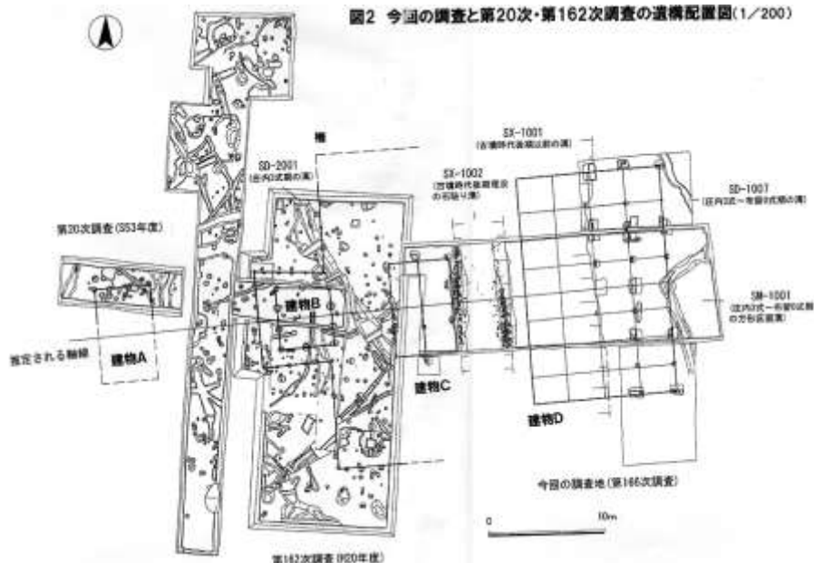
図2 今回の調査と第20次・第162次調査の遺構配置図(1/200)
